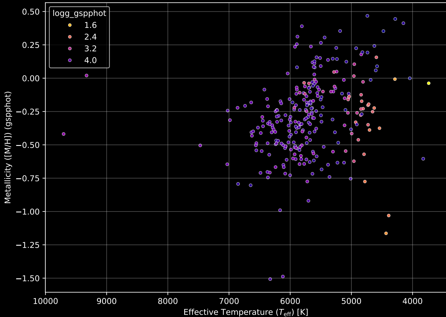
GALAH DR4 Field: [1550] Stellar Population Parameters (n= 273)
